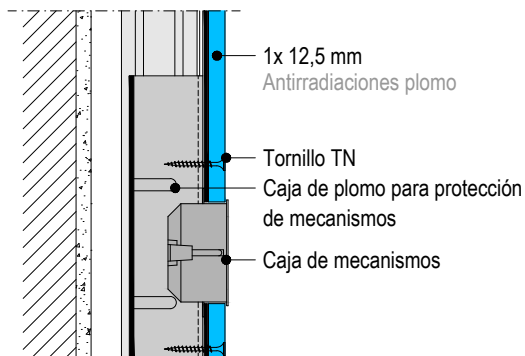
K152B.es-SO1 Caja de mecanismos Sección vertical
