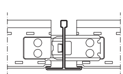
Perfil secundario T 24/32 (15/34) longitud 600 mm
